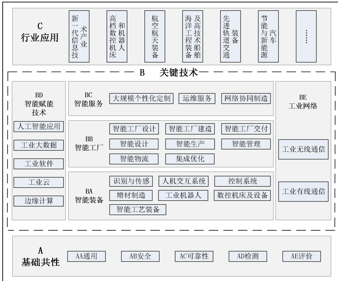
图 2 智能制造标准体系结构图
